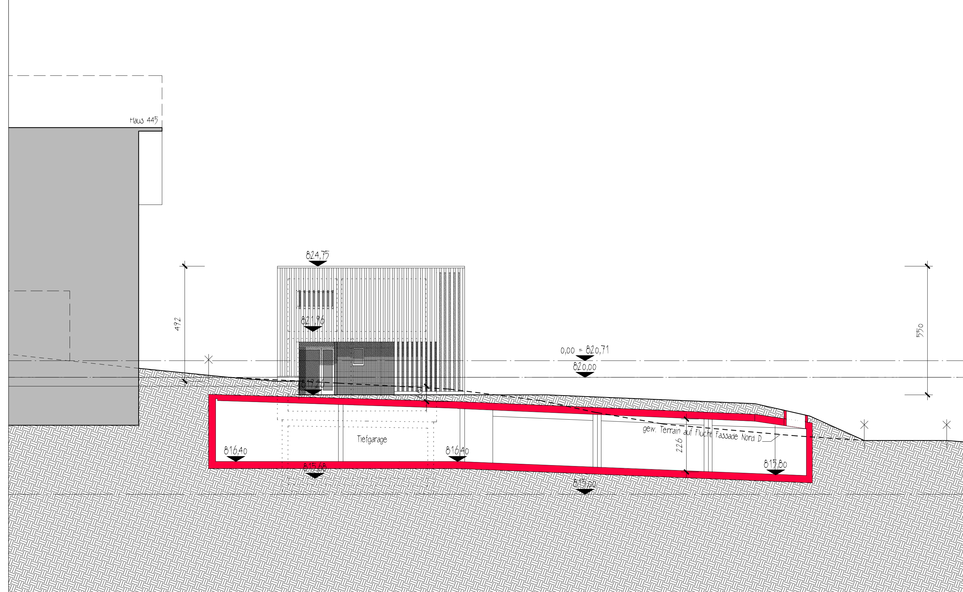
Fassade Süd
