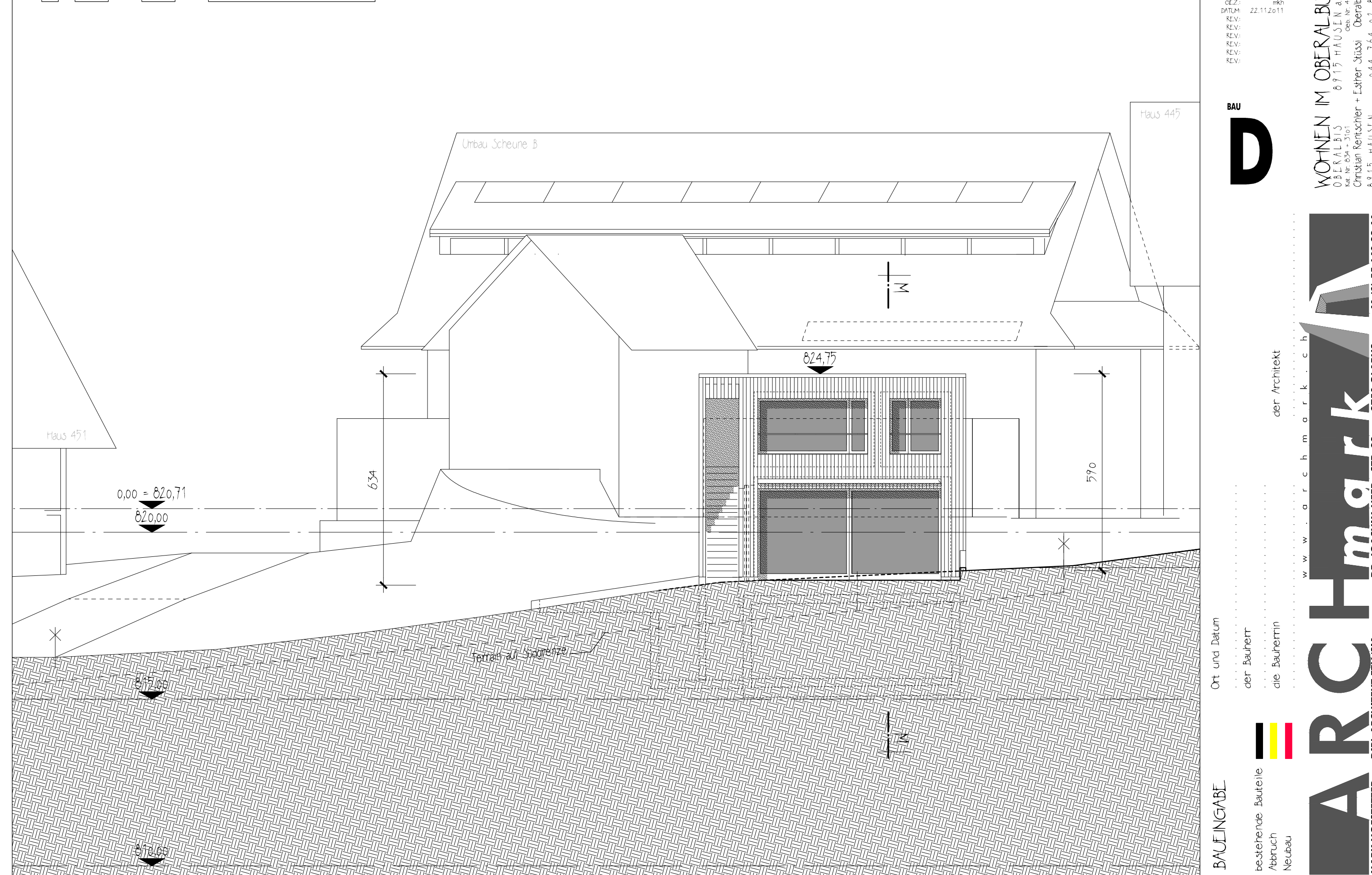
Fassade Süd
